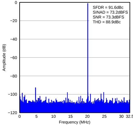
图 48. FFT for 20-MHz Input Signal
