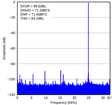
图 49. FFT for 170-MHz Input Signal
