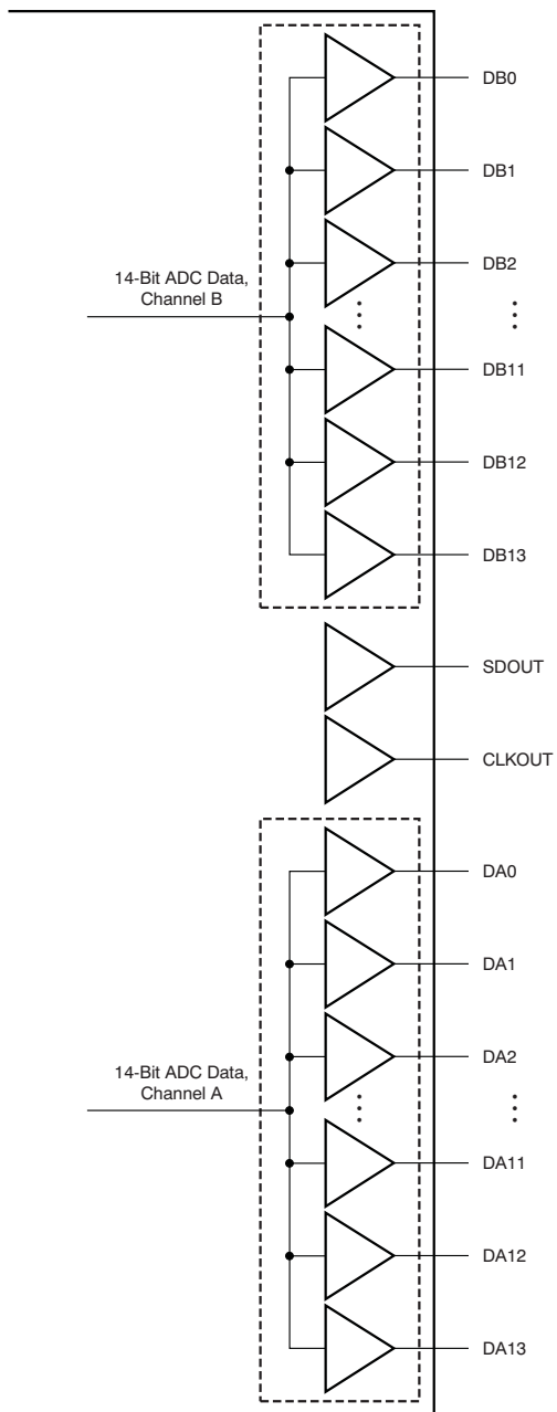
图 158. CMOS Outputs
