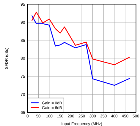
图 109. SFDR vs Input Frequency
