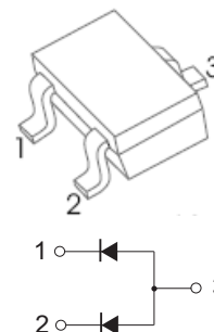
SOT-323
