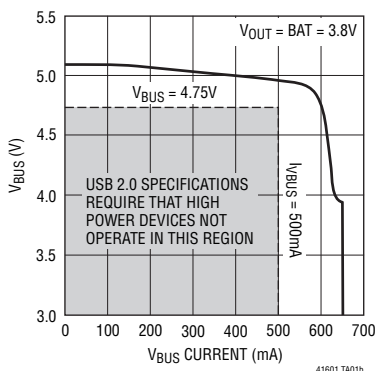
USB OTG V_{BUS} Voltage vs V_{BUS} Current
