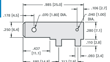
.250 (6.4) TAB
