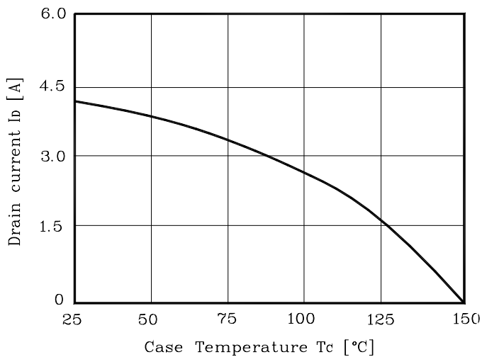
Fig. 9 I_D - T_C
