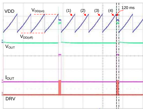
图 28. Soft-Short Protection
