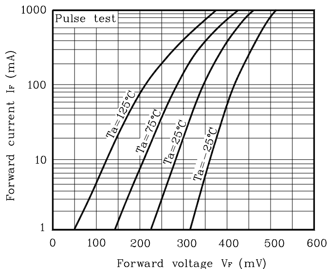
Fig. 1 I_F - V_F
