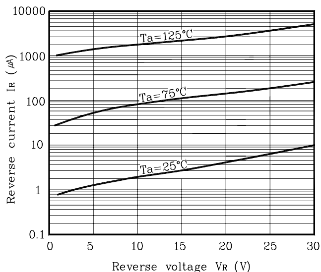
Fig. 2 I_R - V_R
