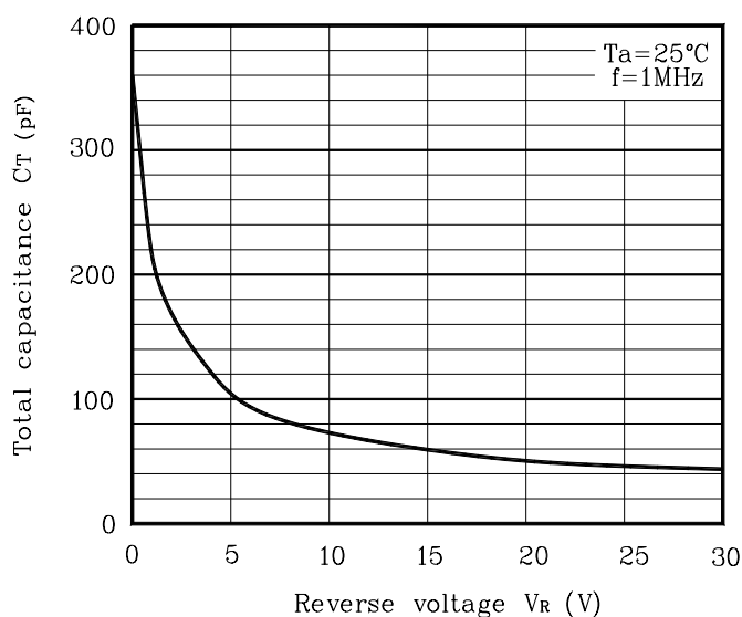
Fig. 3 C_T - V_R
