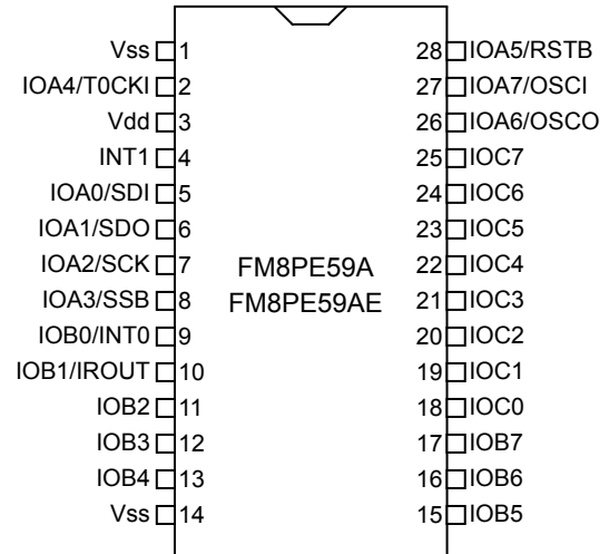
SSOP
