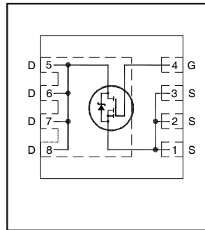
3.3mm x 3.3mm PQFN
