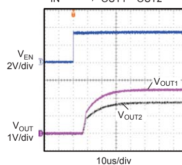
EN Start Up Waveform
