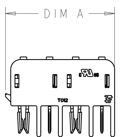
2213614-2/ 1-2213614-2 SCALE 3:1
