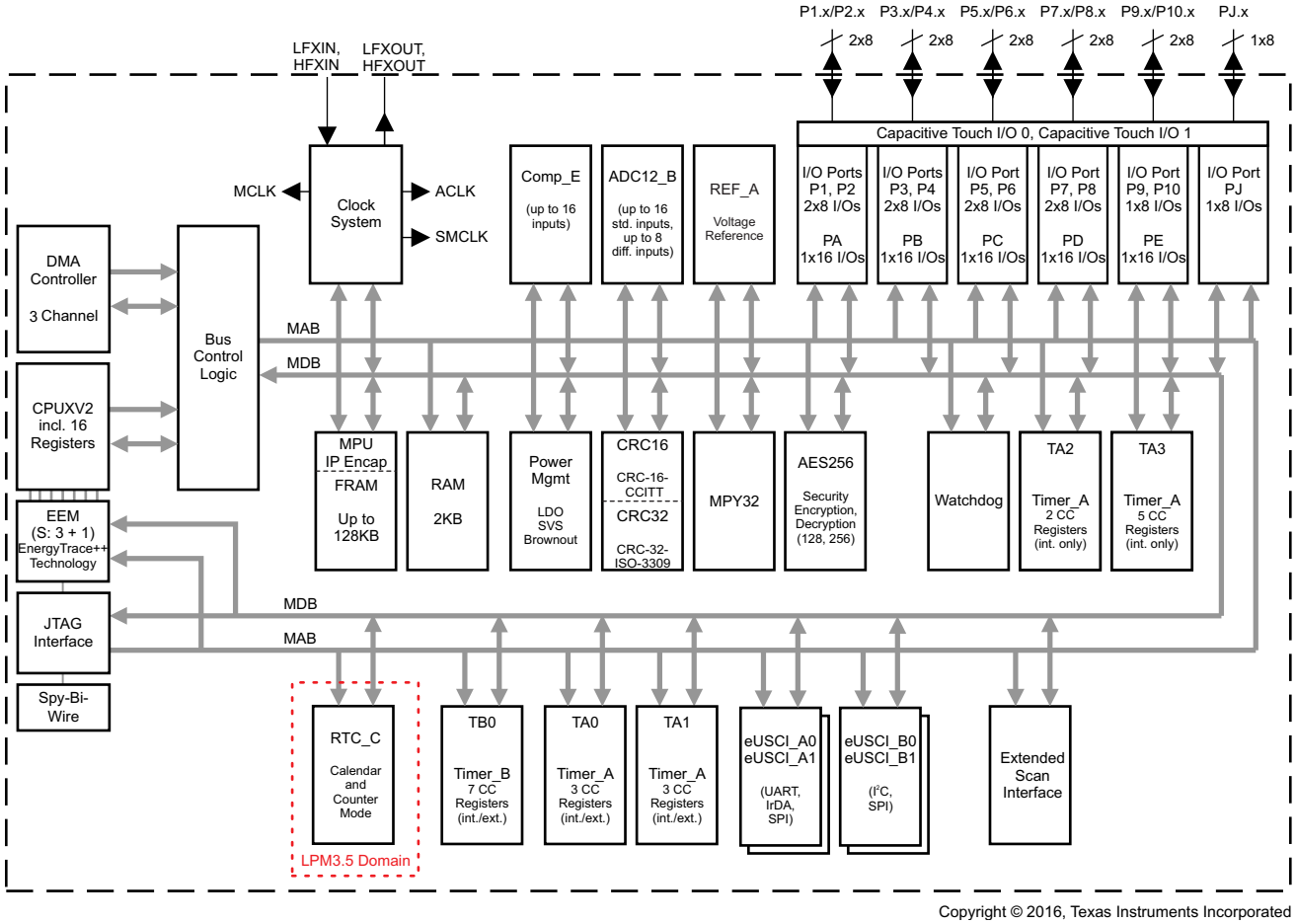
图 1-2. 功能方框图 – MSP430FR598x、MSP430FR598x1
