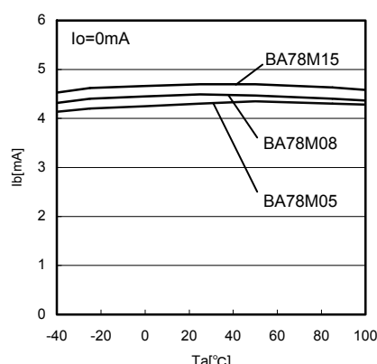
Fig.11 T_a - I_b
