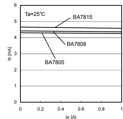
Fig.24 I_o - I_b
