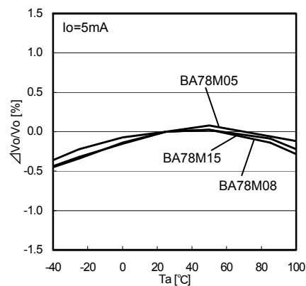
Fig.10 T_a - V_o
