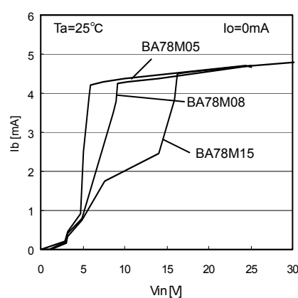
Fig.4 V_{in} - I_b
