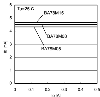
Fig.12 I_o - I_b
