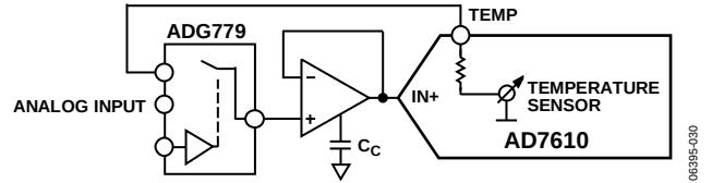
图30. 使用温度传感器
