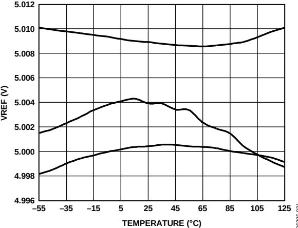
图21. 典型基准电压输出与温度的关系(3个器件)
