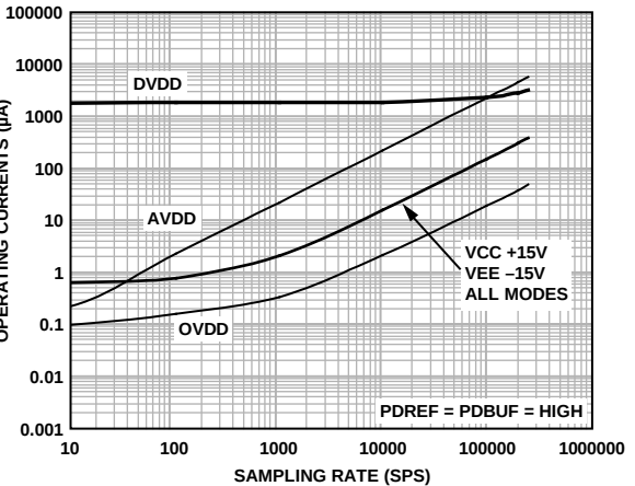
图22. 工作电流与采样速率的关系
