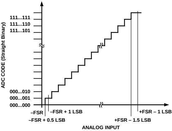
图26. ADC理想传递函数
