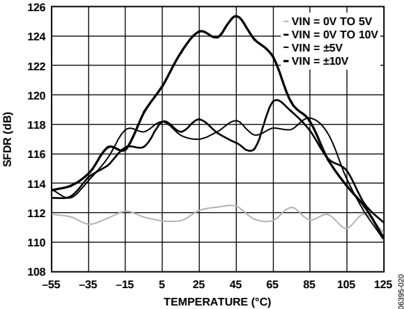
图20. 无杂散动态范围与温度的关系(谐波除外)
