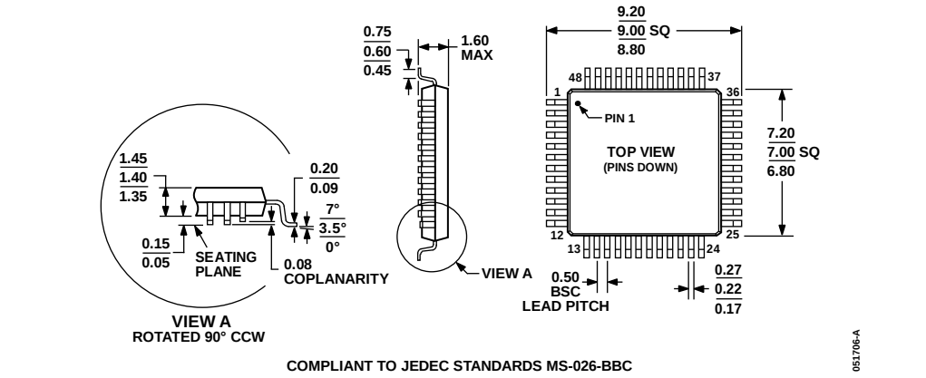
图47. 48引脚LQFP封装(ST-48) 尺寸单位: mm
