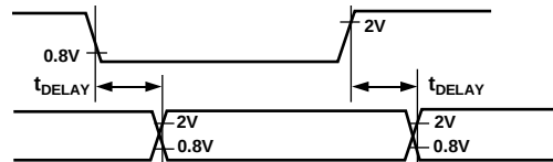
图3. 用于确定时序的基准电平
