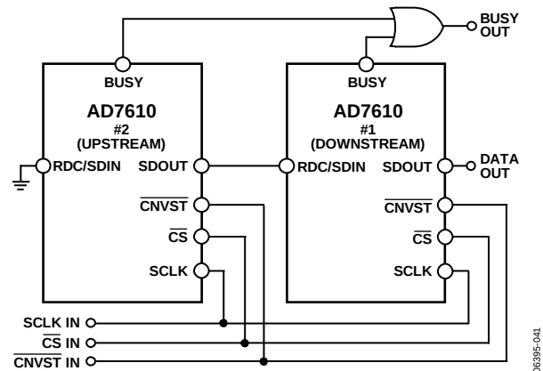
图41. 采用菊花链配置的两个AD7610器件
