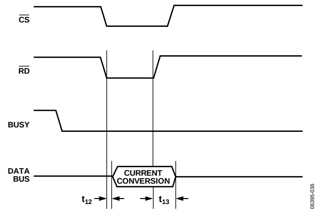
图36. 读取时的从机并行数据时序(转换之后读取)
