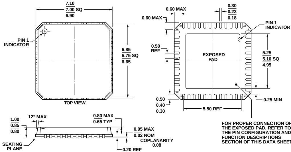
图48. 48引脚引脚架构芯片级封装[LFCSP_VQ] 7 mm × 7 mm, 超薄体 (CP-48-1) 图示尺寸单位: mm
