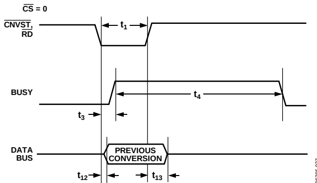
图37. 读取时的从机并行数据时序(转换期间读取)
