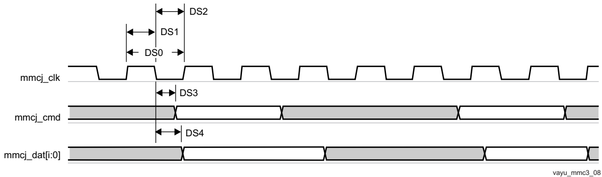
图 7-82. MMC/SD/SDIOj in - Default Speed - Transmitter Mode
