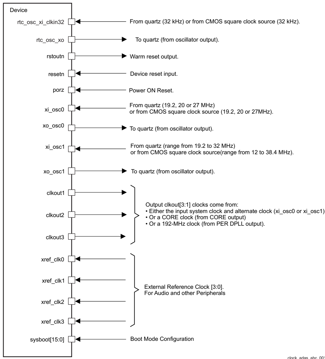
图 6-1. Clock Interface
