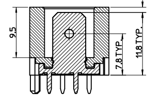
A-A Scale 3:1
