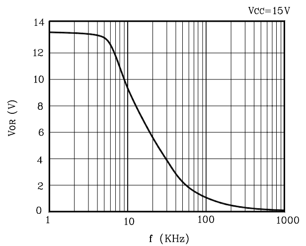
Fig. 4 V_{OR}-f
