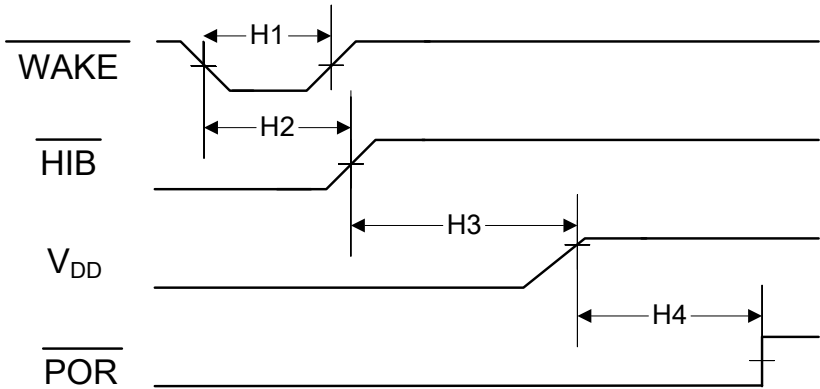
图 23-15. Hibernation Module Timing
