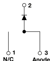
TO-263AB (D²PAK)
