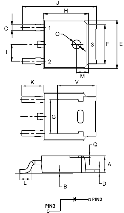
(TO-252) DPAK
