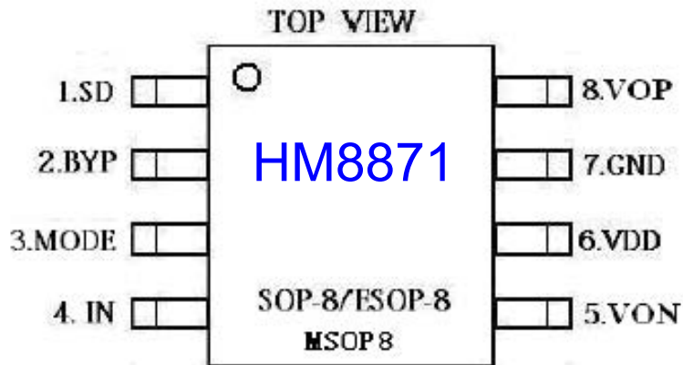
HM8871 SOP8、ESOP8、MSOP8.封装的管脚分布图
