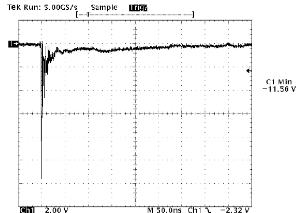
Fig6 - ESD Clamping (-8KV Contac per IEC61000-4-2)
