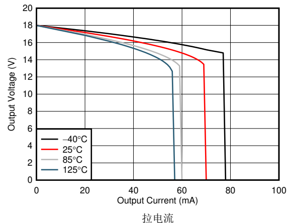
图 6-18. 输出电压摆幅与输出电流间的关系
