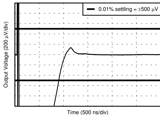
图 6-43. 0.01% 稳定时间
