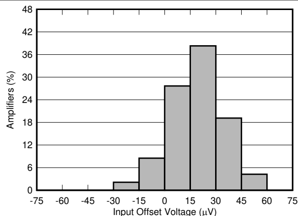
图 6-4. 失调电压生产分配
