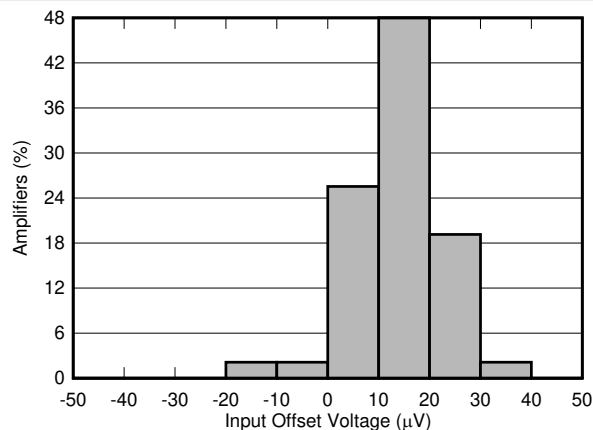
图 6-2. 失调电压生产分配
