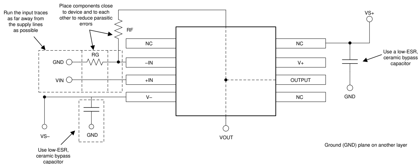
图 11-2. 同相配置的运算放大器电路板布局
