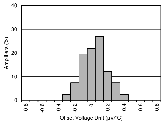
图 6-8. 失调电压漂移分配
