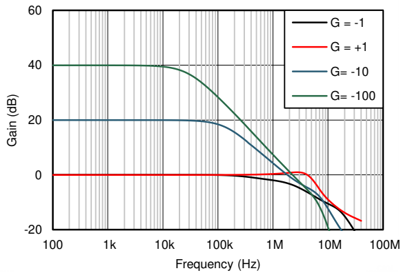
图 6-15. 闭环增益与频率间的关系
