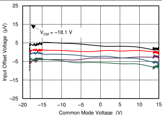
图 6-11. 失调电压与共模电压间的关系
