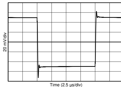
图 6-34. 无相位反转
