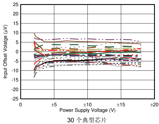
图 6-13. 失调电压与电源间的关系
