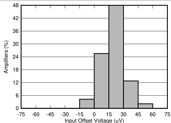
图 6-3. 失调电压生产分配
