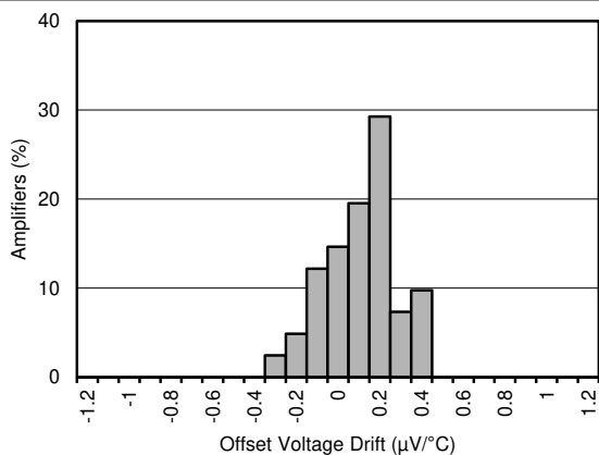
图 6-7. 失调电压漂移分配
