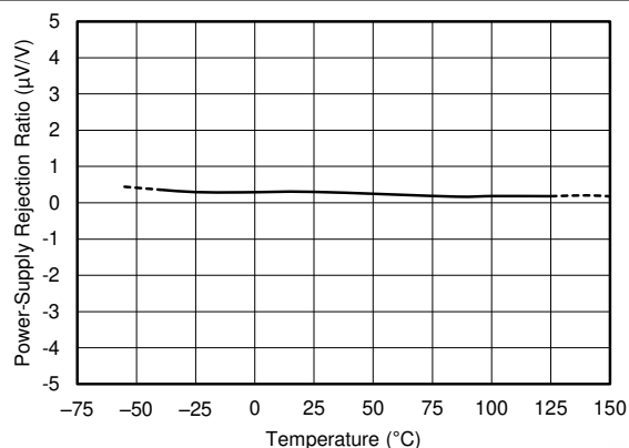
图 6-22. PSRR 与温度间的关系
