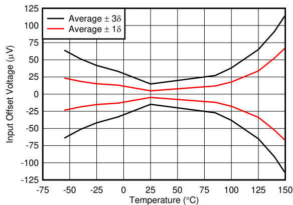
图 6-7. 失调电压漂移分配
