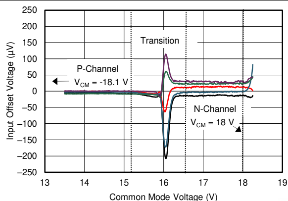
图 6-12. 失调电压与共模电压间的关系 (转换区域)
