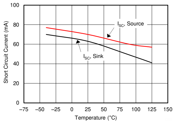
图 6-44. 短路电流与温度间的关系
