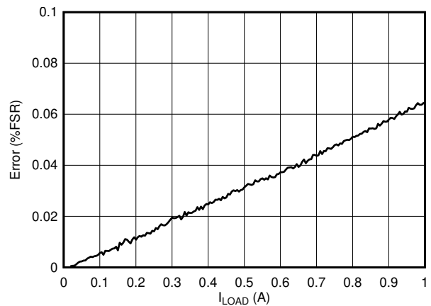
图 9-3. 低侧电流感测满量程误差
