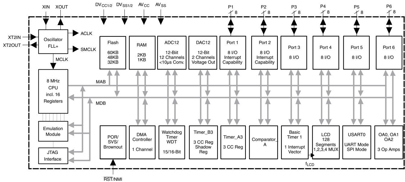
功能方框图
