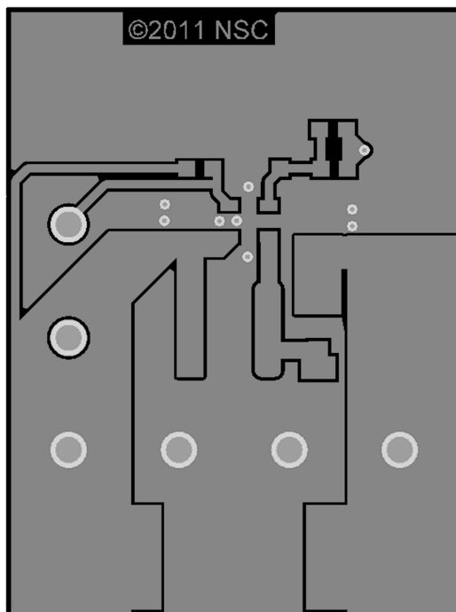
Top Layer
