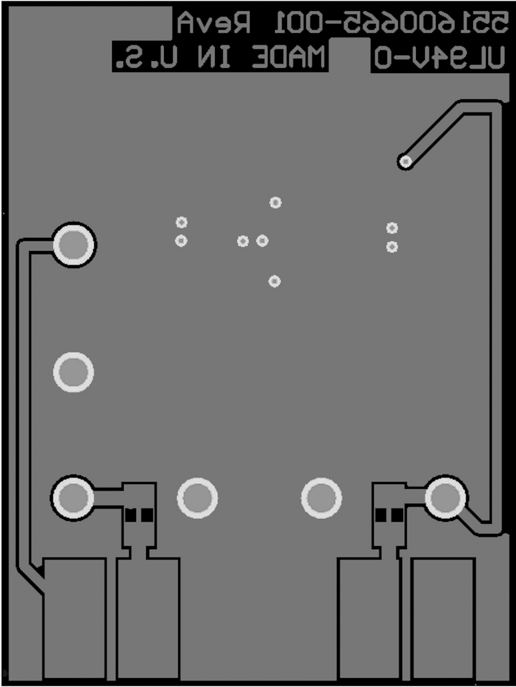
Bottom Layer
