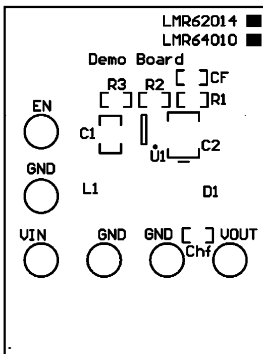
Top Overlay
