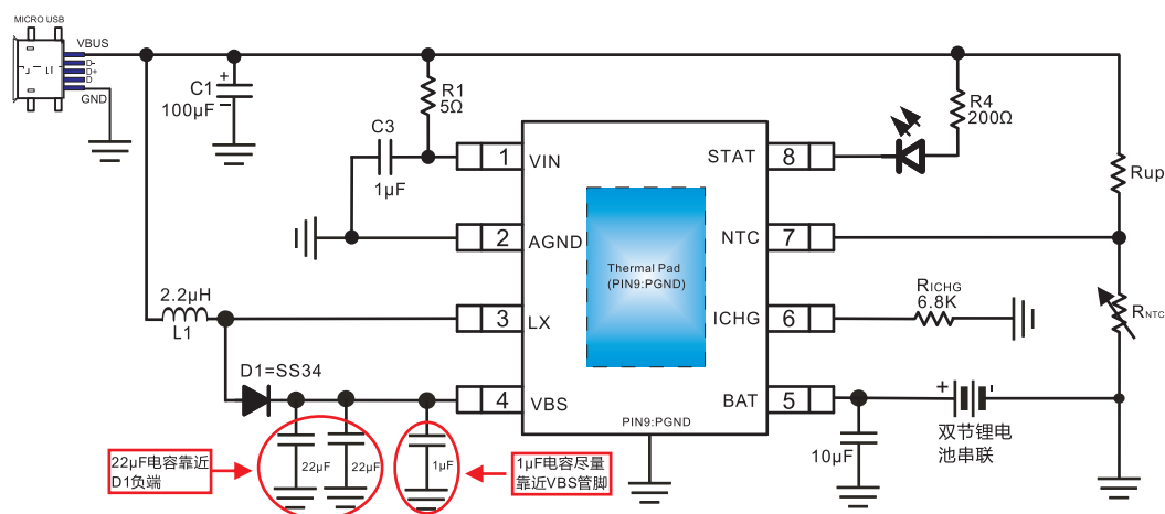
CS5082E应用电路图
