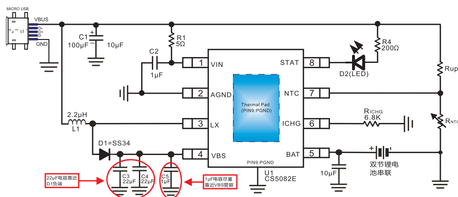
CS5082E充电线路图
