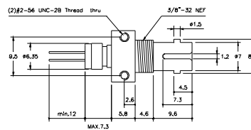
ST Receptacle
