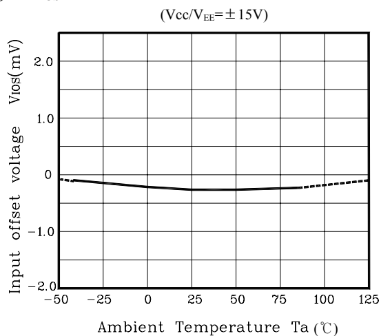
Fig. 9 V_{IOS} - T_a
