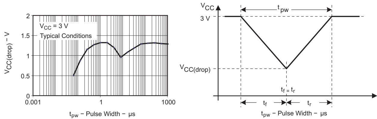
Figure 11. 具有一个三角形压降的 V_{CC} (压降) 电平用于生成一个 POR / 欠压信号
