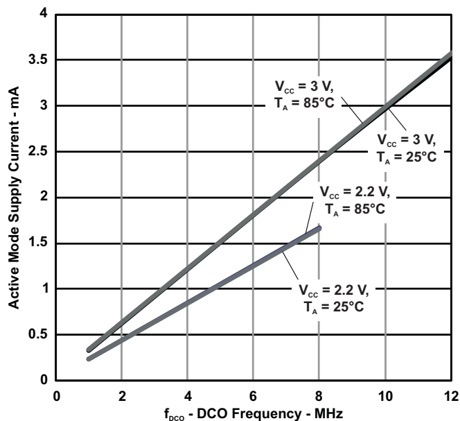
Figure 3. 有源模式电流与 DCO 频率间的关系
