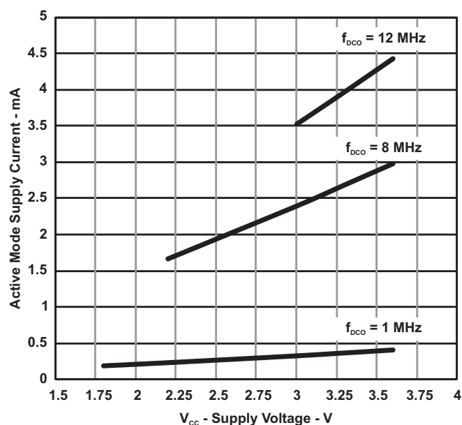
Figure 2. 有源模式电流与 V_{CC} 间的关系, T_A=25^{\circ}C
