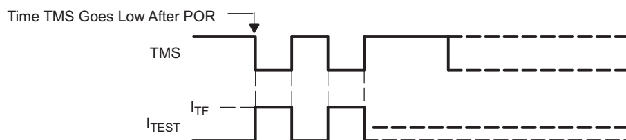
Figure 17. 熔丝检查模式电流
