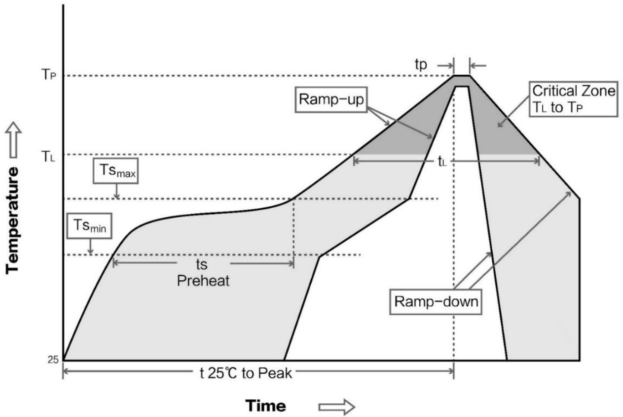
图表 十一-2 回流焊曲线图
