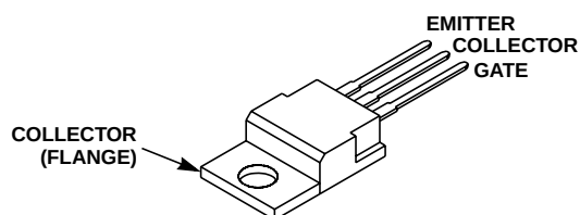
JEDEC TO-220AB
