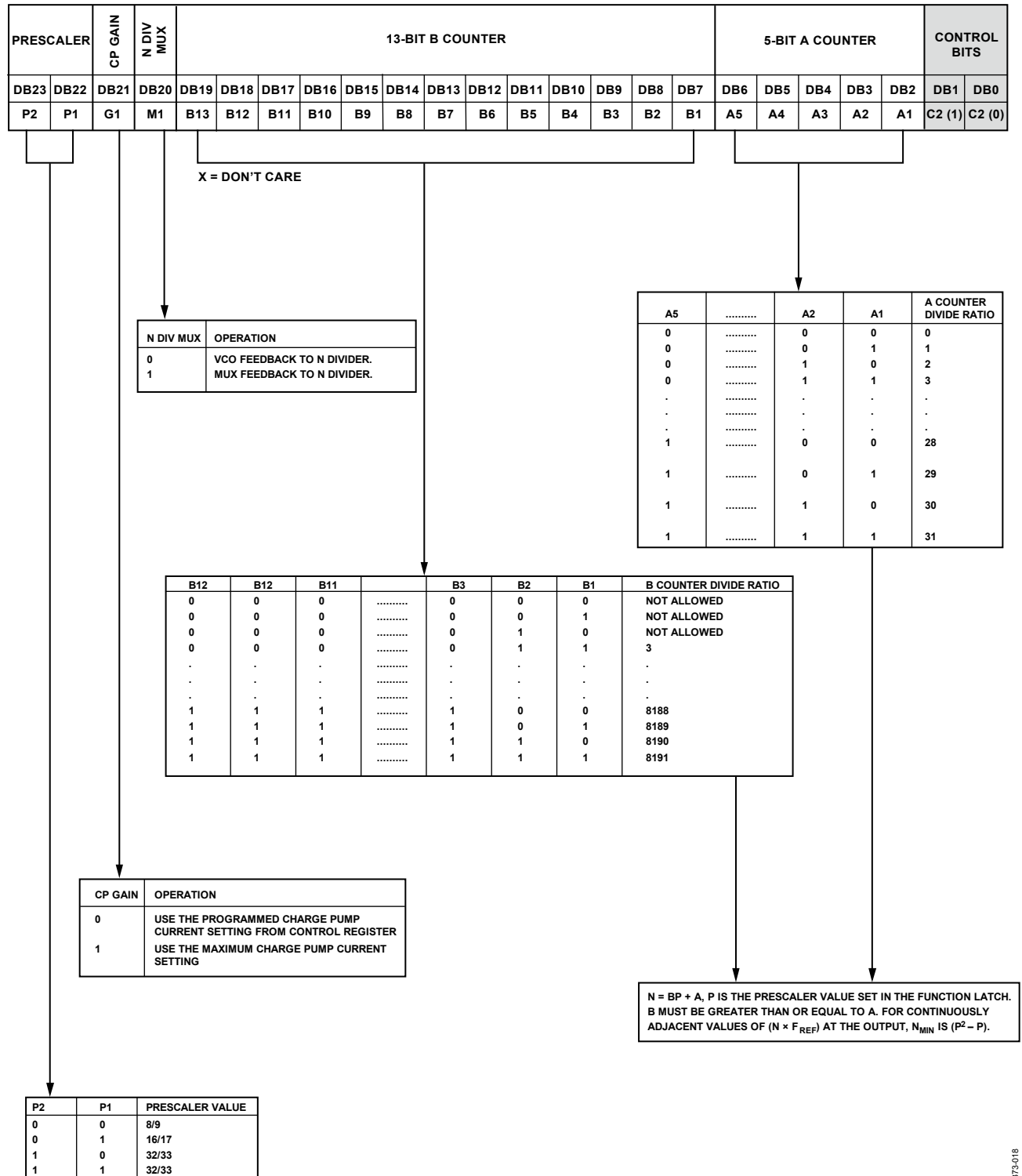
Figure 25. LO Latch
