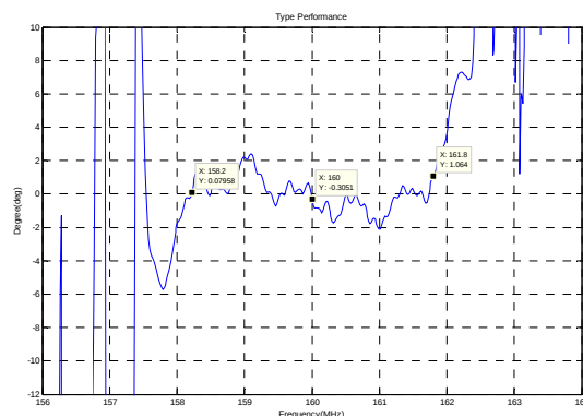
Phase Linearity( f_0 \pm 1.8\text{MHz} )
