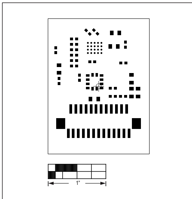
MAX86140OSBEK#—Top Paste
