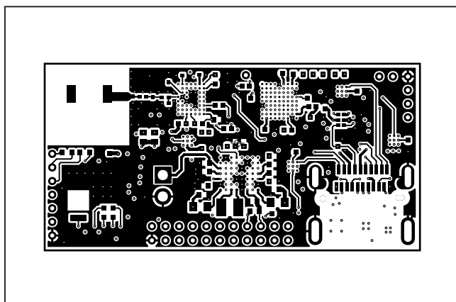
MAX32620UCBLEEK#—Top
