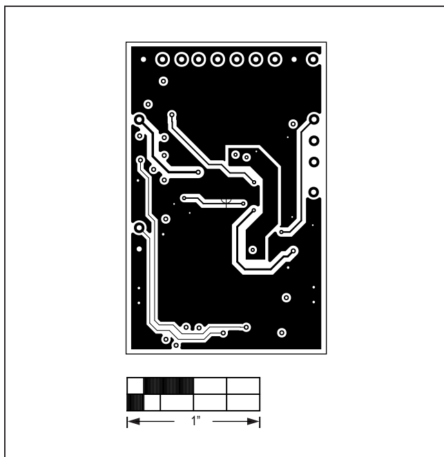
MAX86141OSBEK#—L04 SIG
