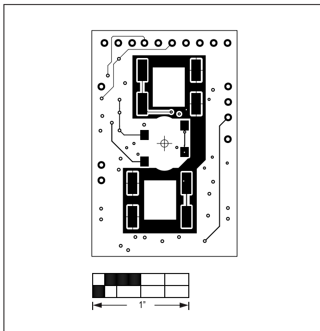
MAX86141OSBEK#—L05 SIG
