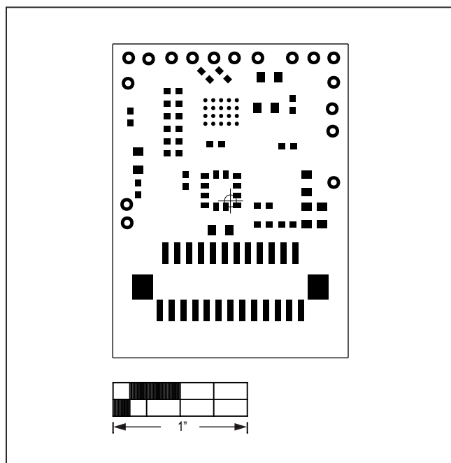
MAX86140OSBEK#—Top Mask
