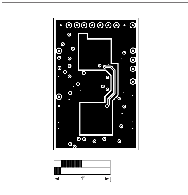
MAX86141OSBEK#—Top
