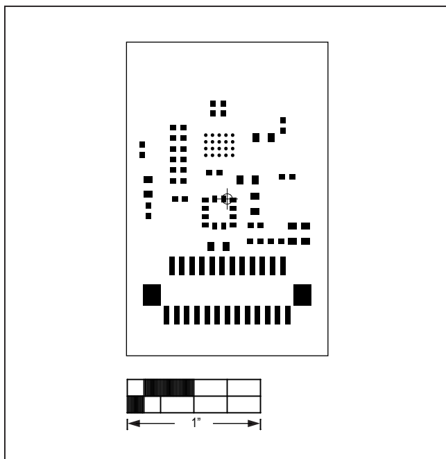
MAX86141OSBEK#—Top Paste
