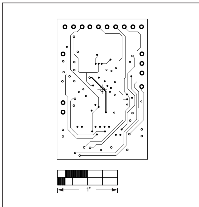
MAX86141OSBEK#—L03 SIG
