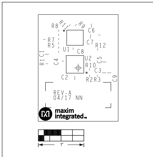
MAX86140OSBEK#—Top Silkscreen
