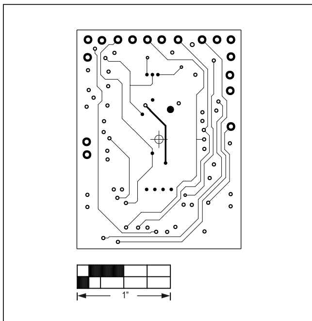
MAX86140OSBEK#—L03 GND
