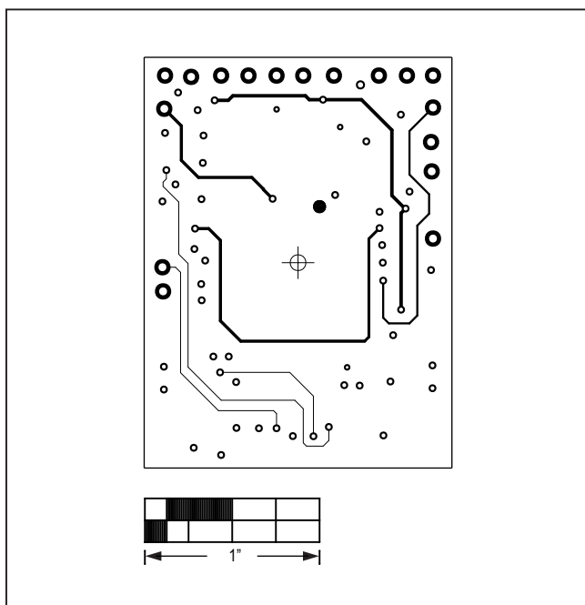
MAX86140OSBEK#—L04 SIG
