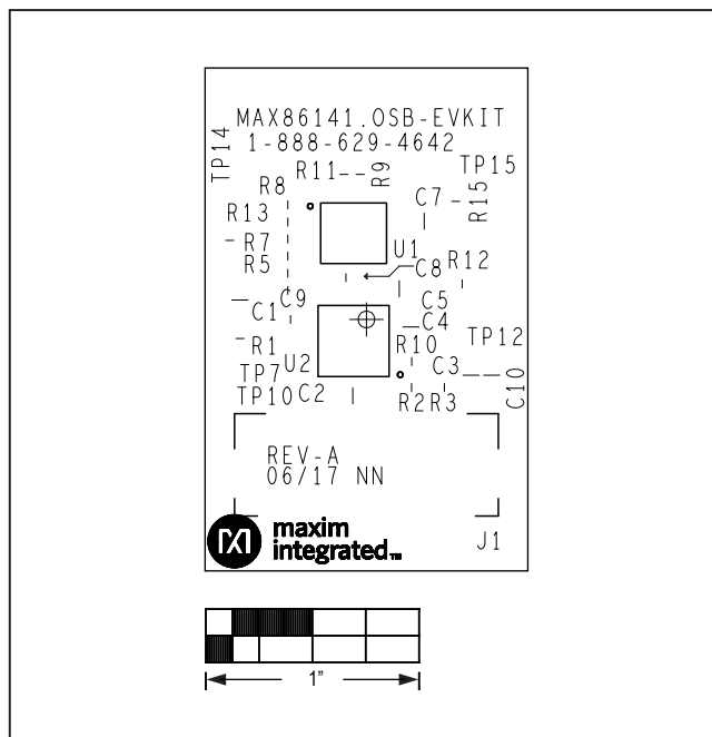
MAX86141OSBEK#—Top Silkscreen
