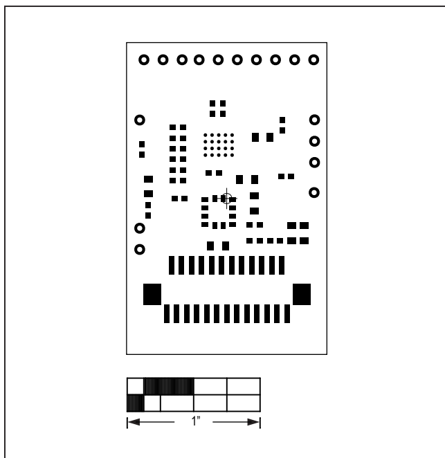
MAX86141OSBEK#—Top Mask
