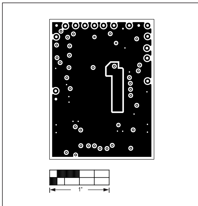
MAX86140OSBEK#—L05 SIG
