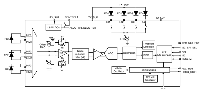
简化方框图
