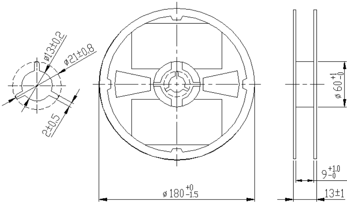
Reel Dimensions
