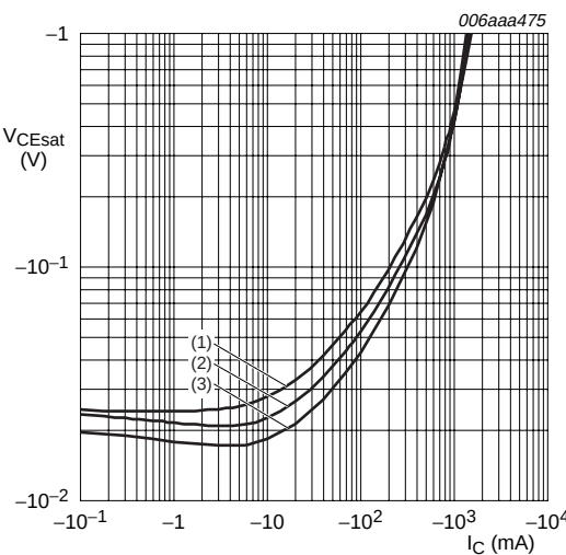
I_C/I_B = 20 (1) T_{amb} = 100 °C (2) T_{amb} = 25 °C (3) T_{amb} = -55 °C
