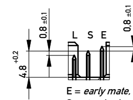
Stecklänge / mating length
