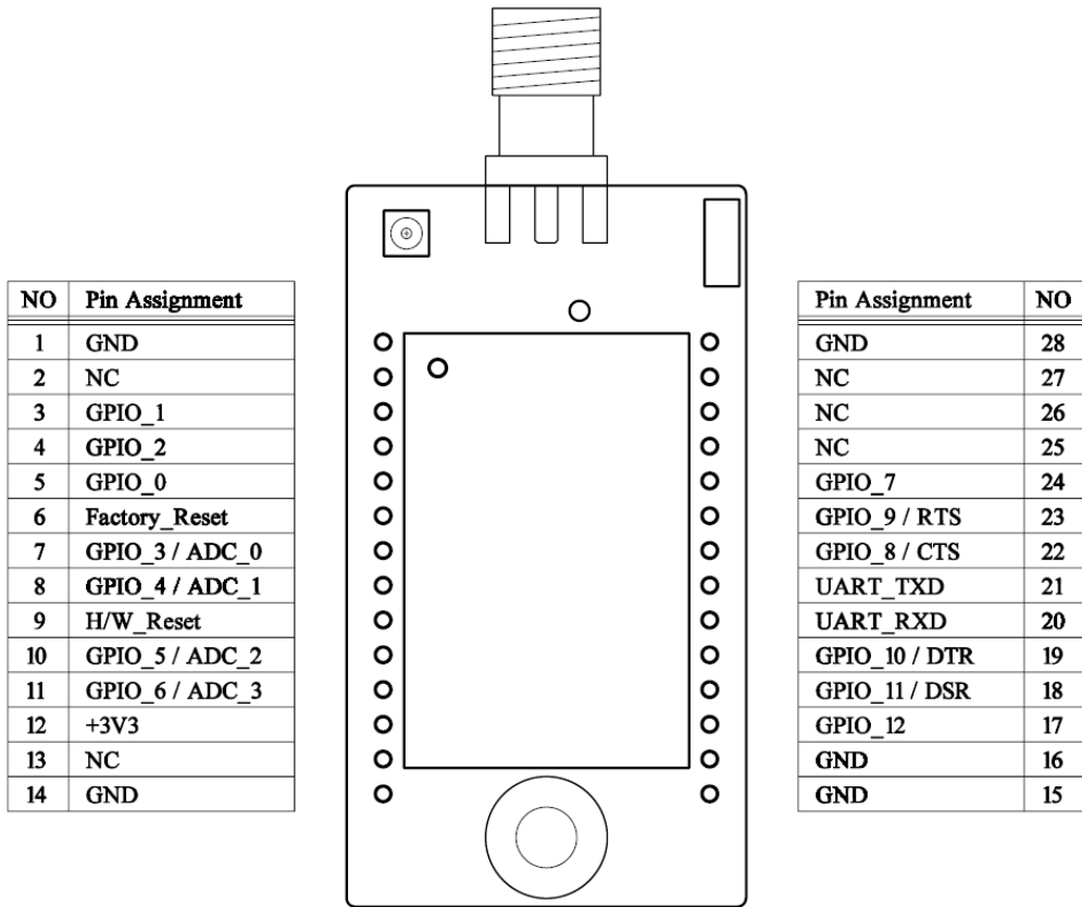
그림 1-2 핀 배치도
