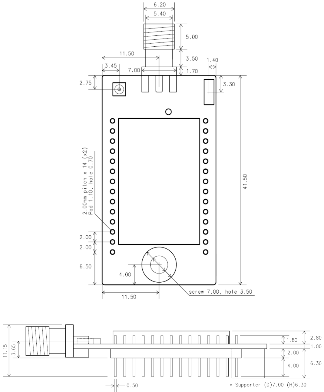
그림 1-3 치수도
