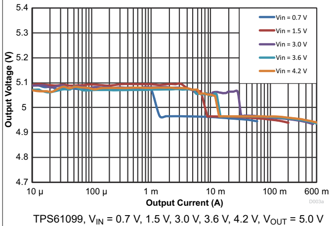
图 7-9. Load Regulation
