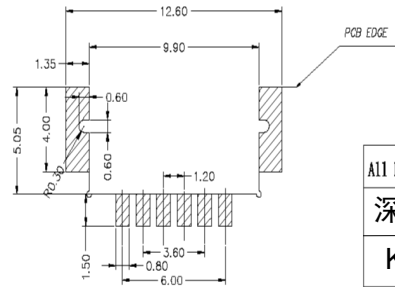
PCB LAYOUT 图仅供参考
