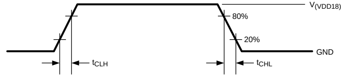
图 1. LVCMOS Transition Times
