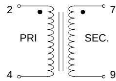
T-30406 & 30408 Schematic
