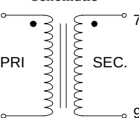
T-30402 & 30403 Schematic
