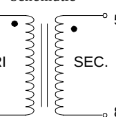
T-30401 Schematic
