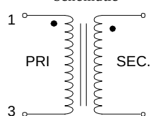
T-30400 Schematic
