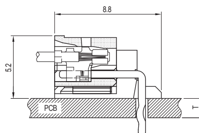
PCB ASS'Y
