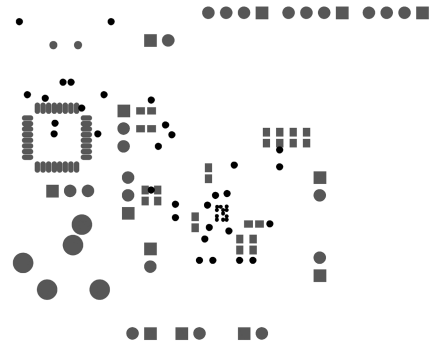
Past Mask Bottom Layer
