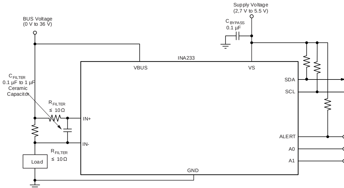
图 25. Input Filtering
