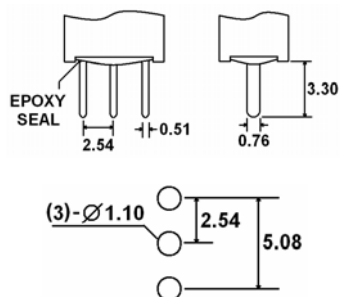
C – SPDT
