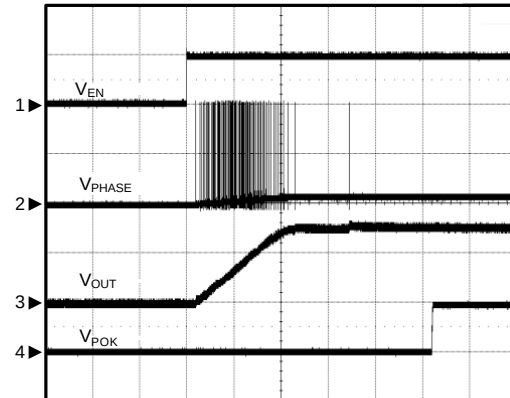
Enable(Auto)
