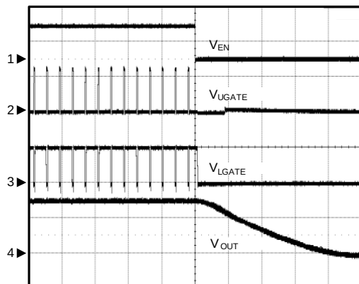
Disable(15A)
