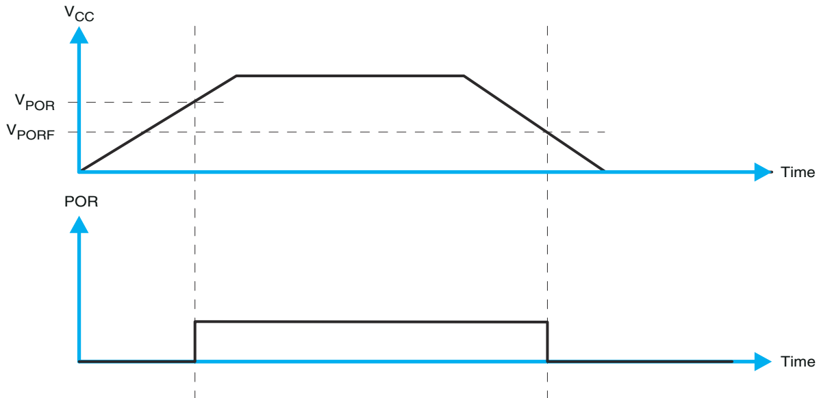
图 10-4. V_{POR}
