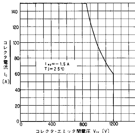
安全動作領域(逆バイアス)
